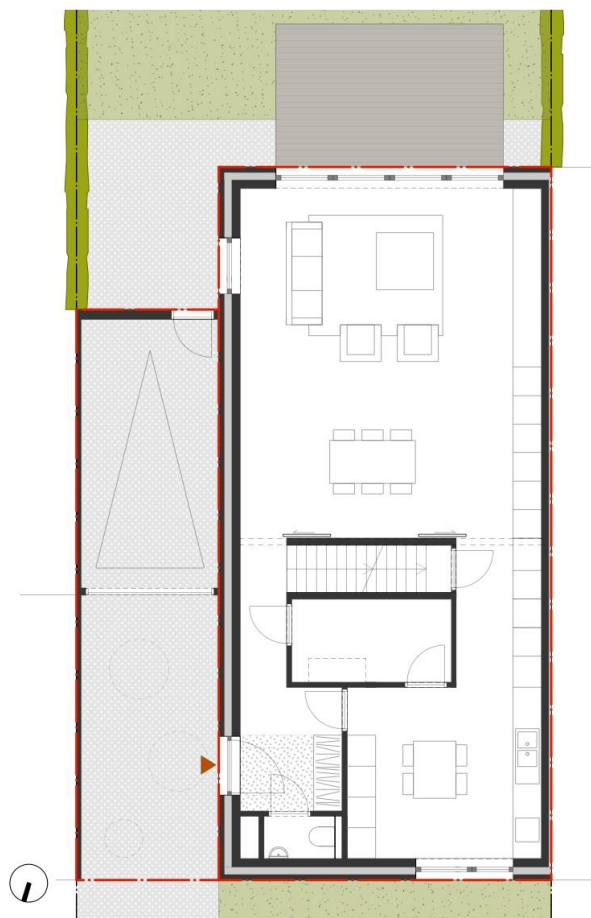
BENEDENVERDIEPING
