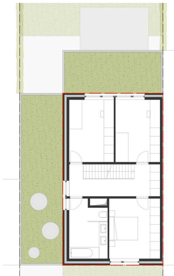
EERSTE VERDIEPING
