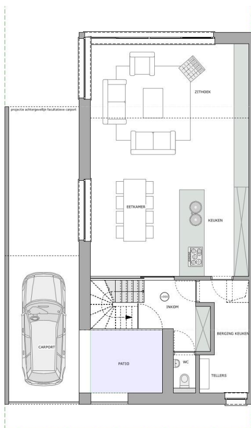
BENEDENVERDIEPING
